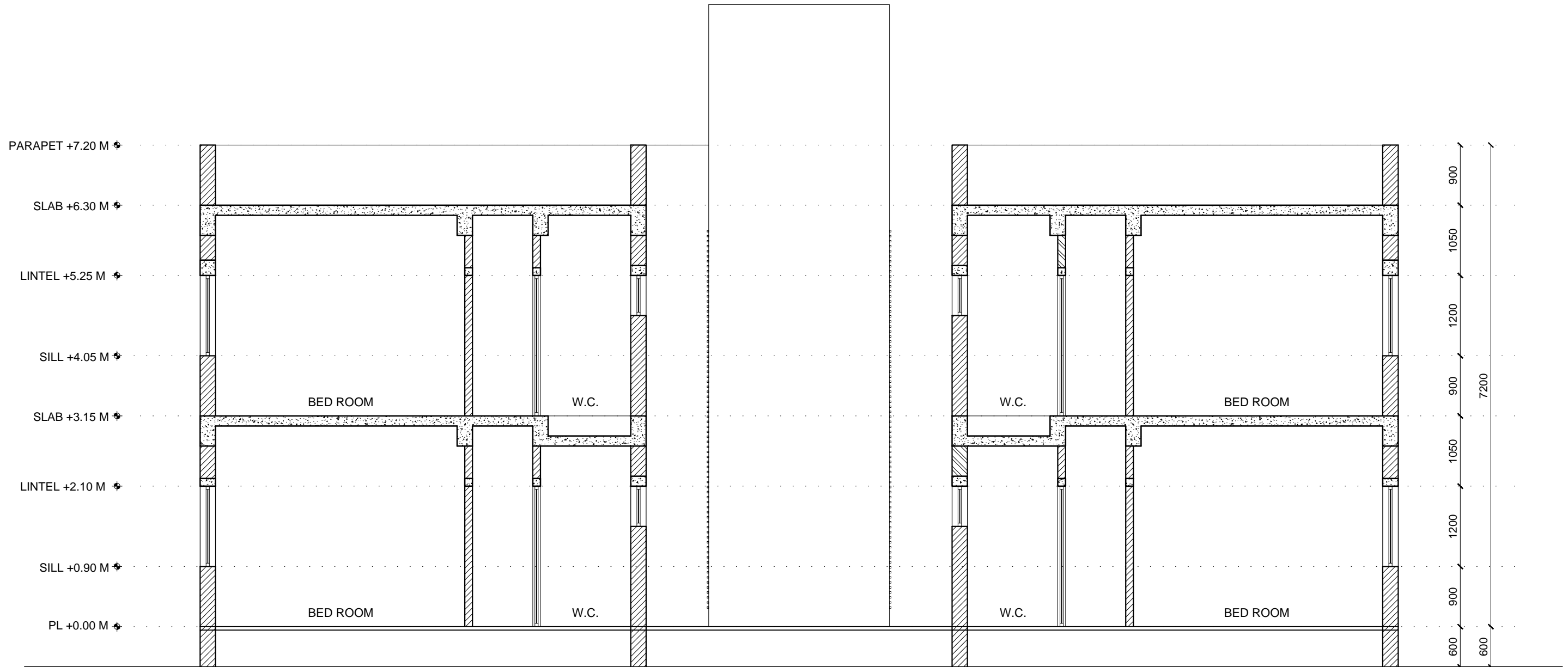
SECTION - D D'
